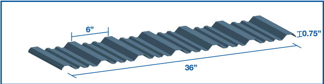
OPTIMUM RIB
