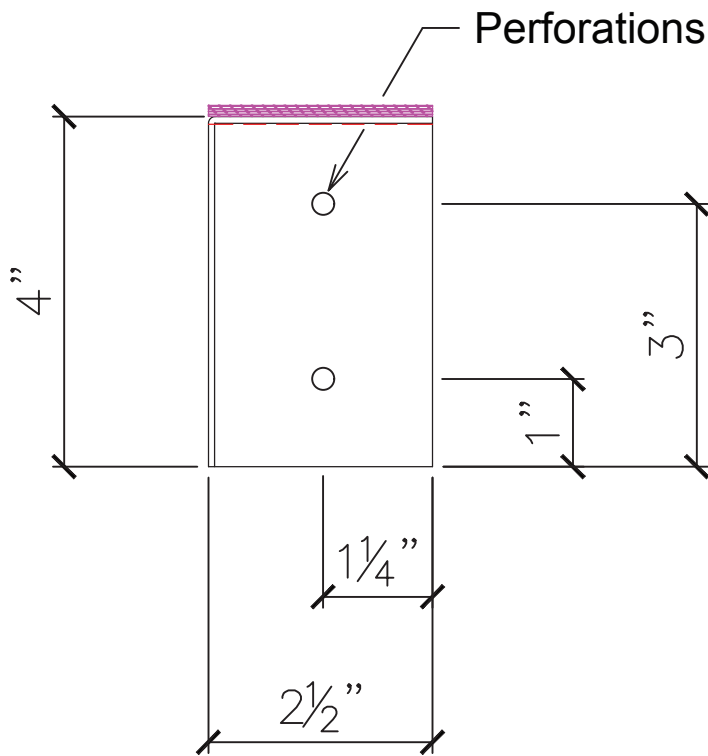
VUE D'AVANT
